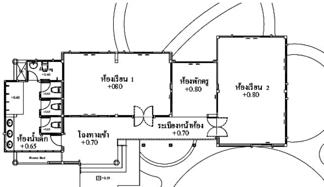
ภาพแสดงผังอาคารเรียนหลังที่ ๒
